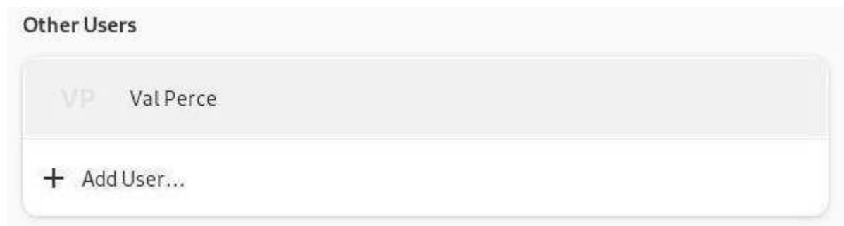
Users list
