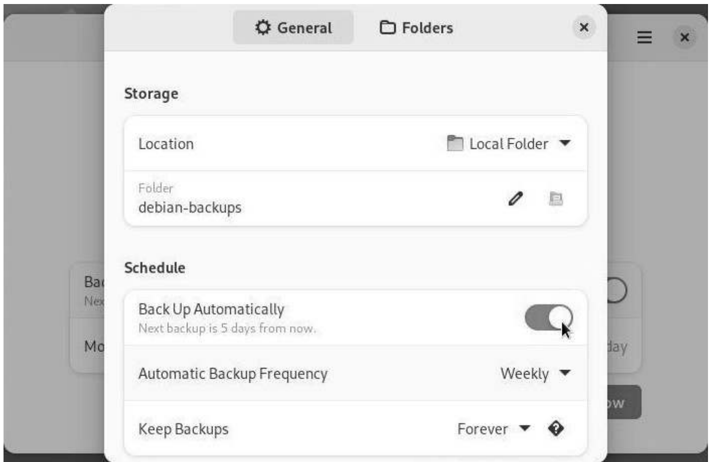
Deja-Dup: preferences
