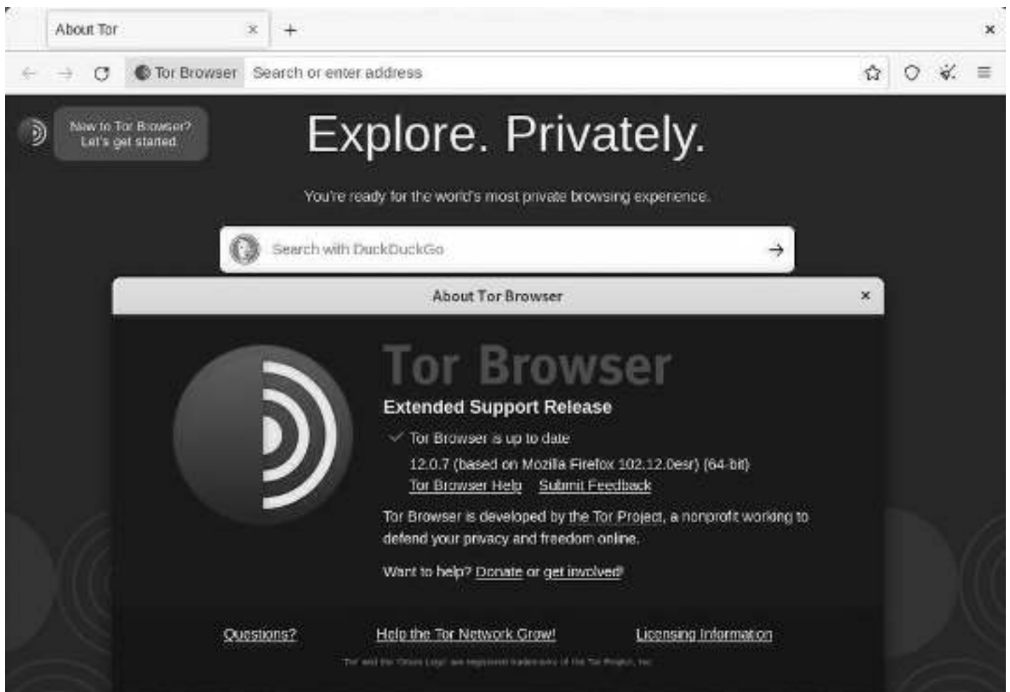
TorBrowser
